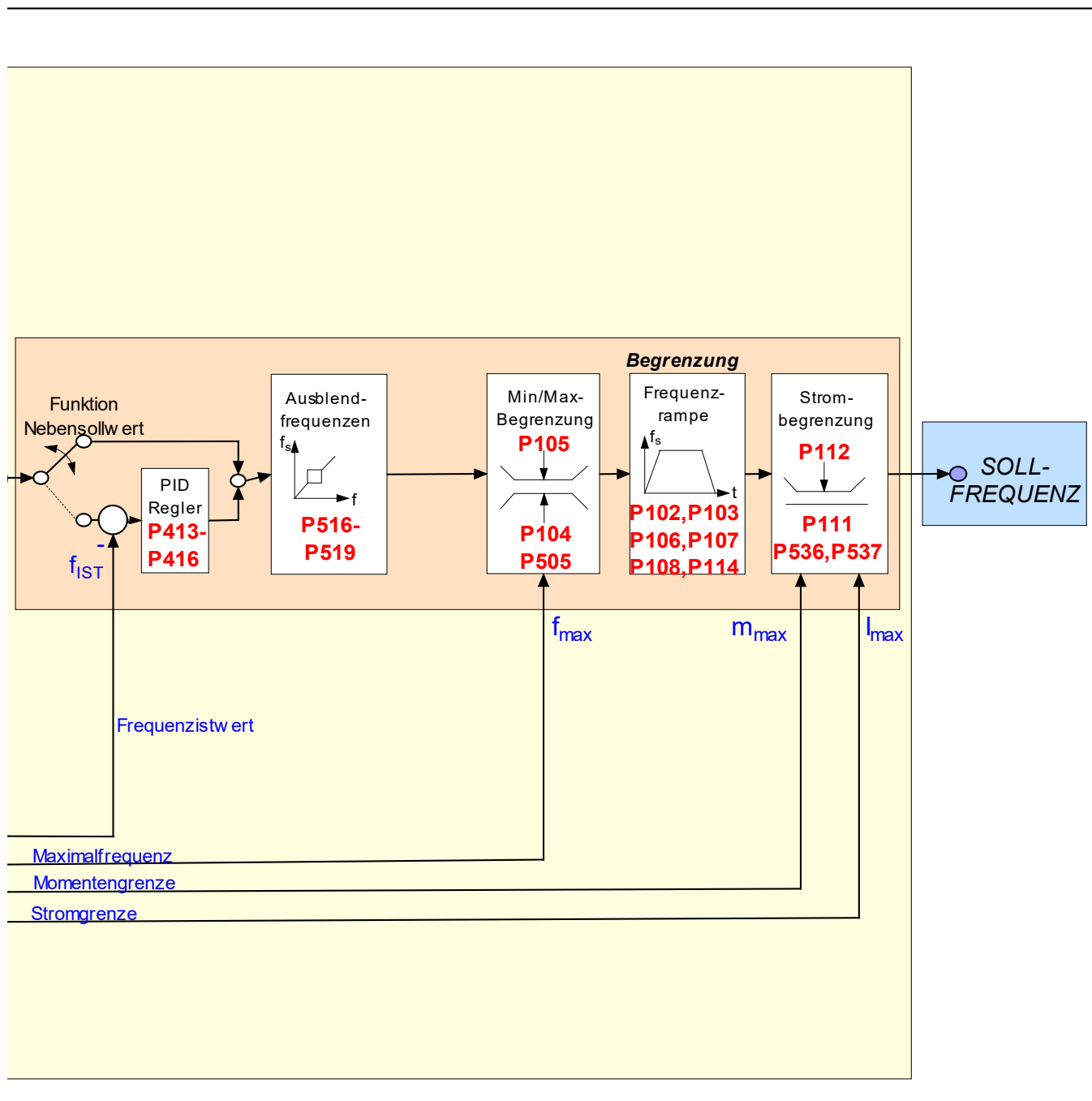
Abbildung 14: Sollwertverarbeitung
