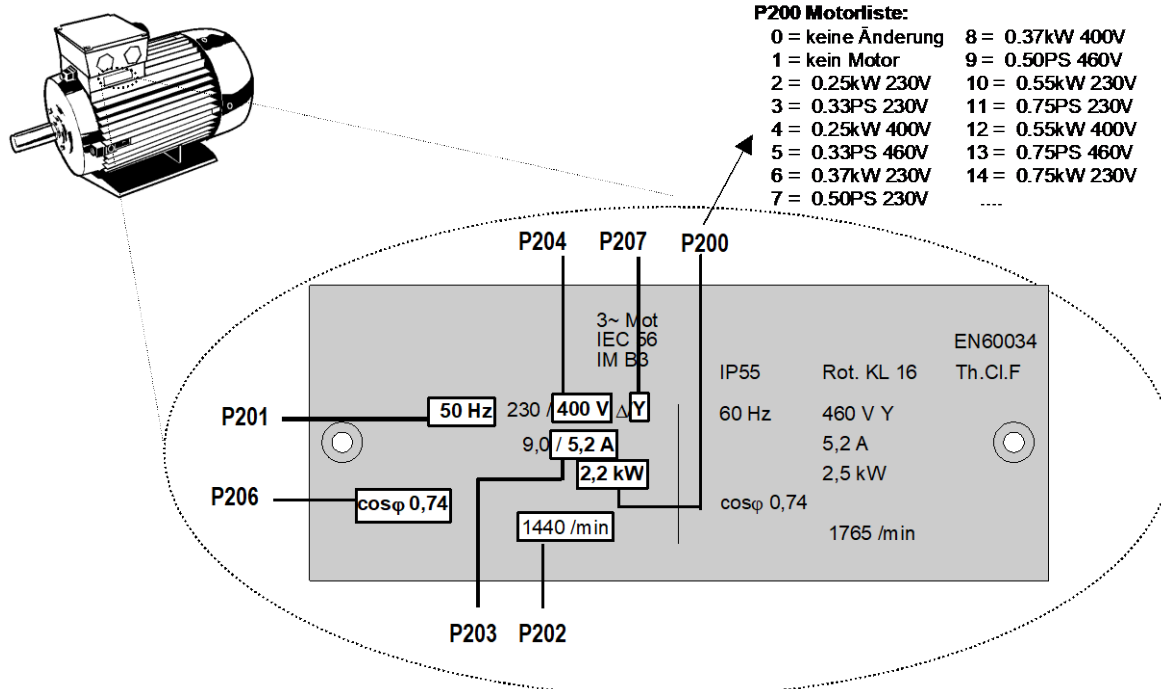
Abbildung 13: Motortypenschild
