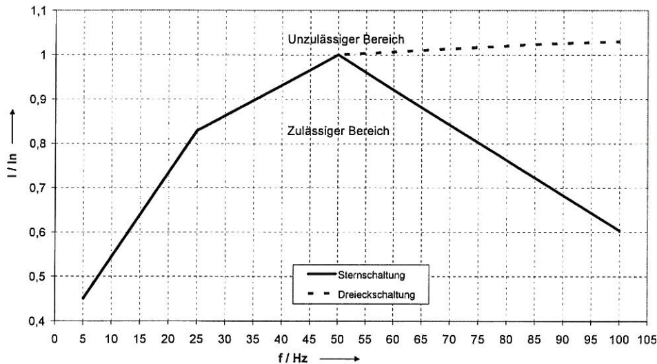
Einstellparameter für die Dauerstromgrenze des Frequenzumrichters zwischen 5 Hz und 100 Hz
