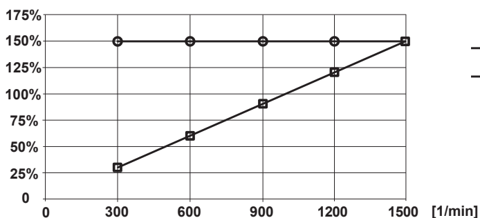
Praca przerywana S3-10%, 1:5, charakterystyka 50 Hz
