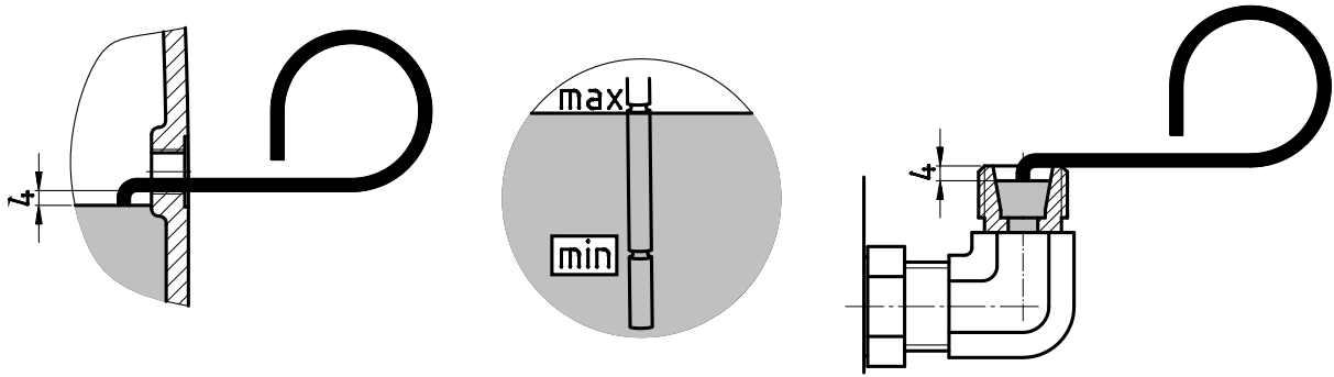
Şekil 27: Yağ ölçüm çubuğuyla yağ seviyesinin kontrol edilmesi
