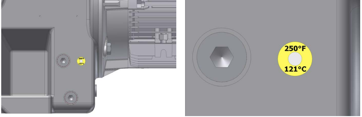
Şekil 20: Sıcaklık etiketinin konumu
