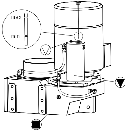
Şekil 37: Yağ seviyesi hazneli paralel milli redüktörler
