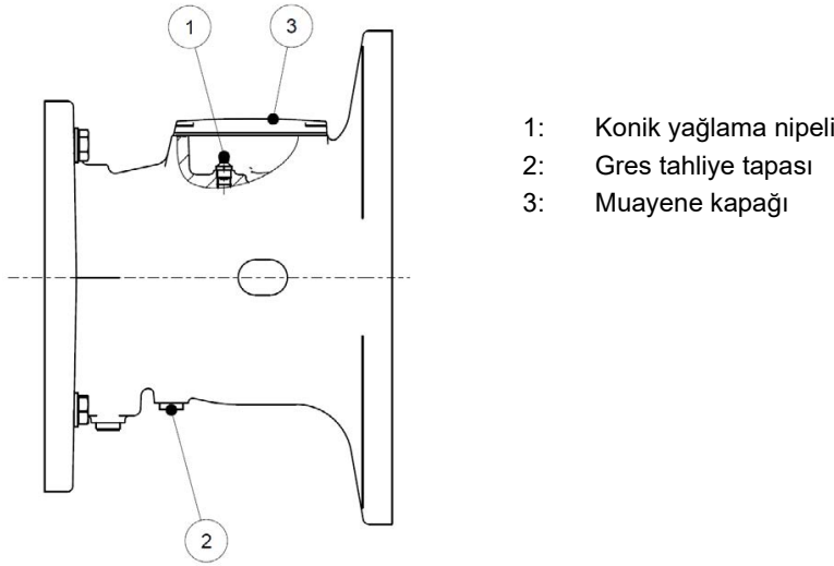
Şekil 31: AI ve AN opsiyon BRG1 IEC/NEMA adaptörünün yağlanması
