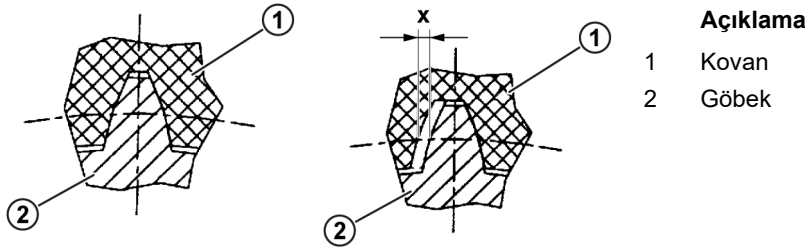
Şekil 30: BoWex® yuvarlak dişli kaplinde dişli kovan aşınmasının ölçülmesi
