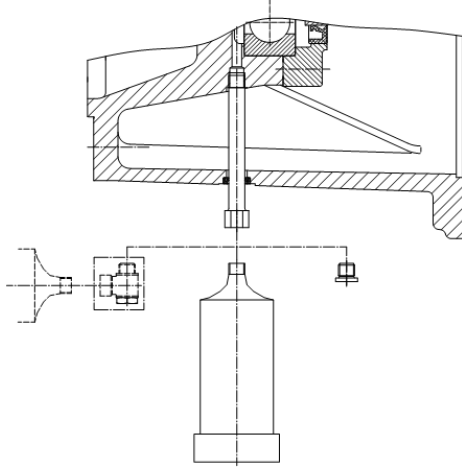
Şekil 22: Gres toplama kabının takılması
