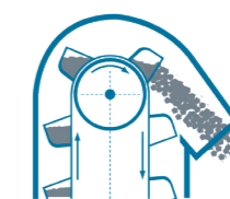
Elevatore centrifugo
