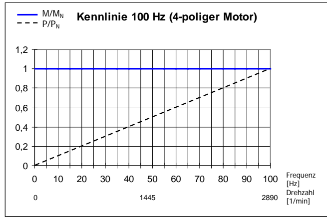
Abbildung 23: Kennlinie 100 Hz
