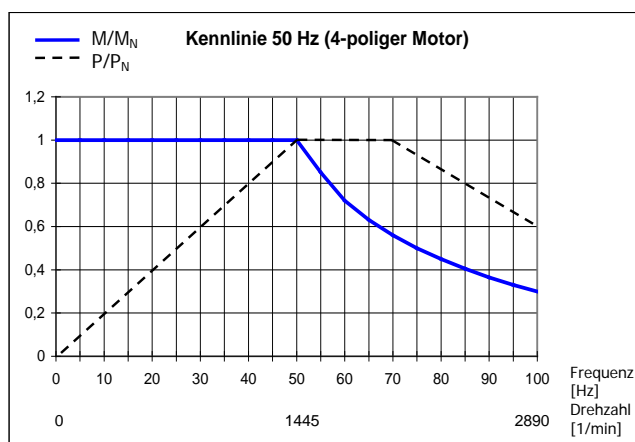
Abbildung 21: Kennlinie 50 Hz
