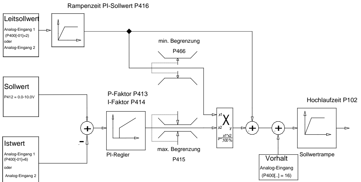
Abbildung 16: Ablaufdiagramm Prozessregler
