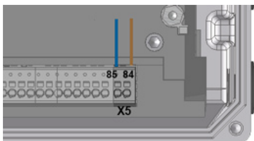
Abbildung 14: Anschlussklemmen AS-i
