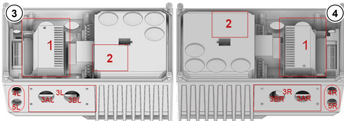
Abbildung 6: Optionsplätze Baugröße 2
