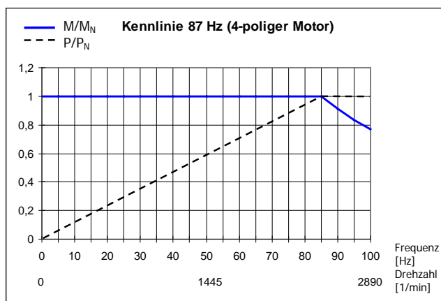
Abbildung 22: Kennlinie 87 Hz
