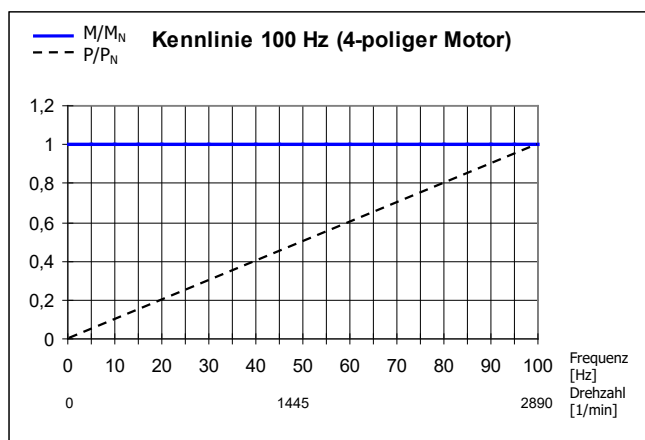
Abbildung 11: Kennlinie 100 Hz
