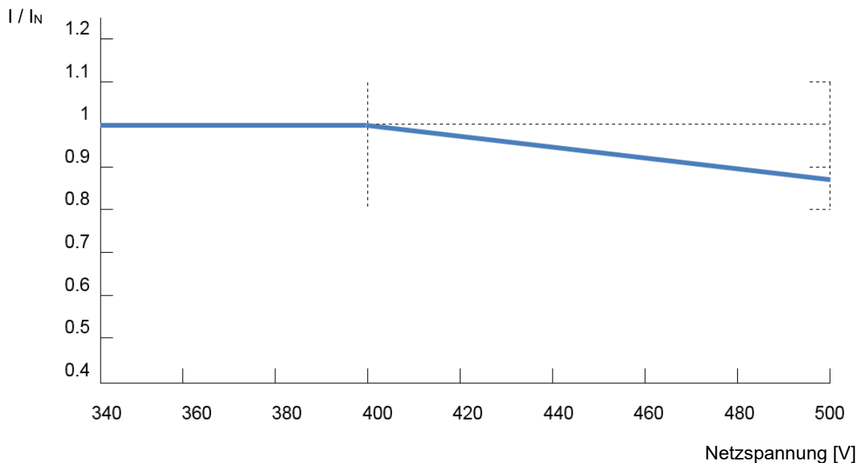
Abbildung 7: Ausgangsstrom aufgrund der Netzspannung
