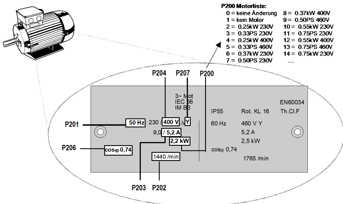
Abbildung 13: Motortypenschild
