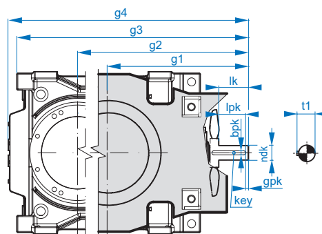
Podwójny pełny wał wyjściowy
