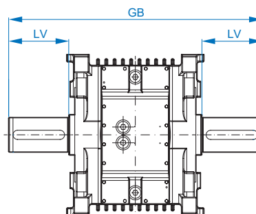
Podwójny pełny wał wyjściowy
