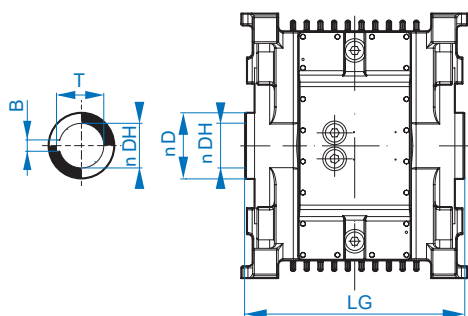
Wał drążony
