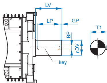
Pełny wał wyjściowy
