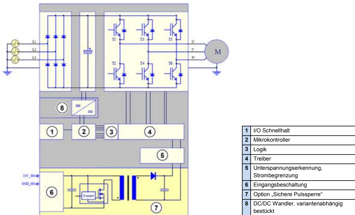
Abbildung 1: Aufbau sichere Pulssperre
