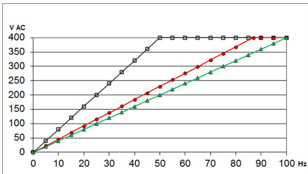
Caratteristiche U/f
