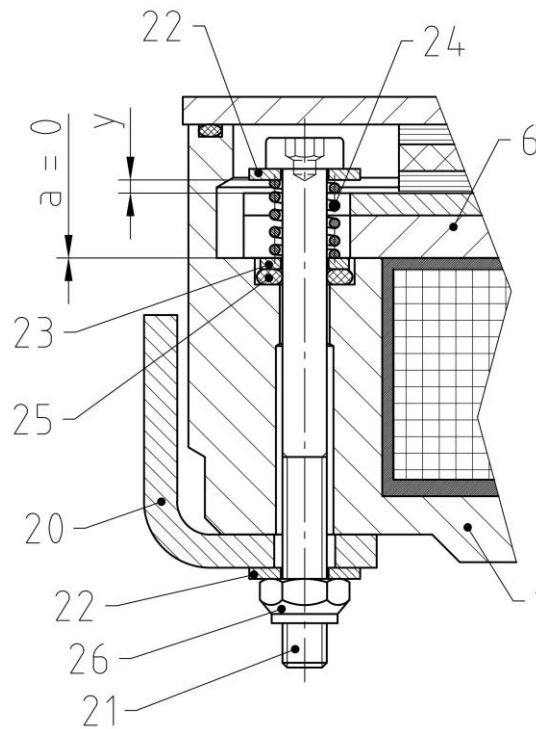
Image 3.2 : Montage / Démontage de la ventilation manuelle (représentation en coupe décalée)
