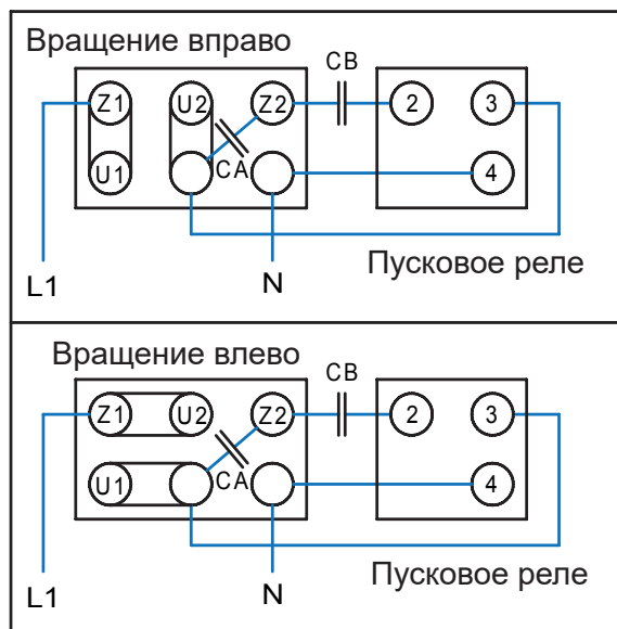
Однофазный электродвигатель ECR NEMA (115 / 230 В) ECR
