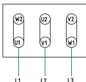
Трехфазный режим Схема «треугольник» \Delta 200 В - 303 В 50 Гц 220 В - 332 В 60 Гц
