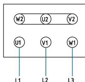
Трехфазный режим Схема «звезда» Y 346 В - 525 В 50 Гц 380 В - 575 В 60 Гц
