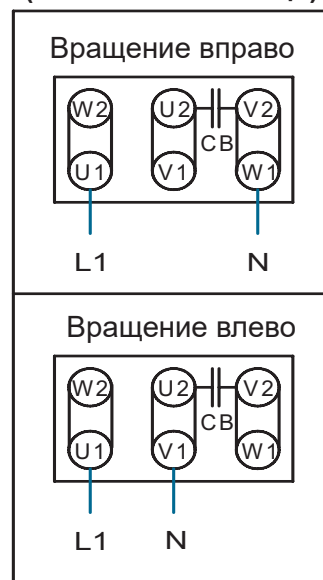
Однофазный электродвигатель EST (схема Штейнметца)
