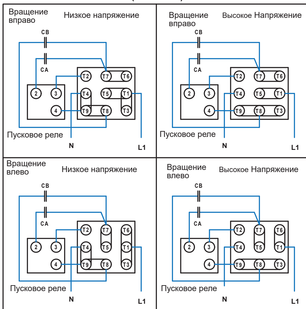
Однофазный электродвигатель ECR NEMA (115 / 230 В) ECR
