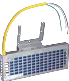
Resistência de travagem externa
