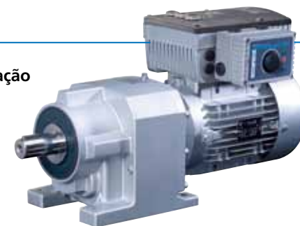
SK 200E com interruptor de manutenção
